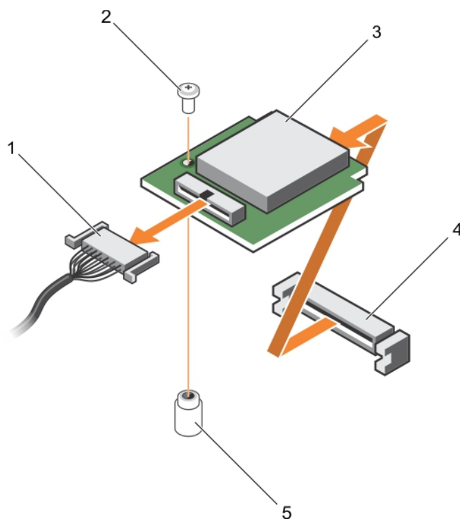
Ilustración 122. Extracción de una unidad de memoria vFlash
