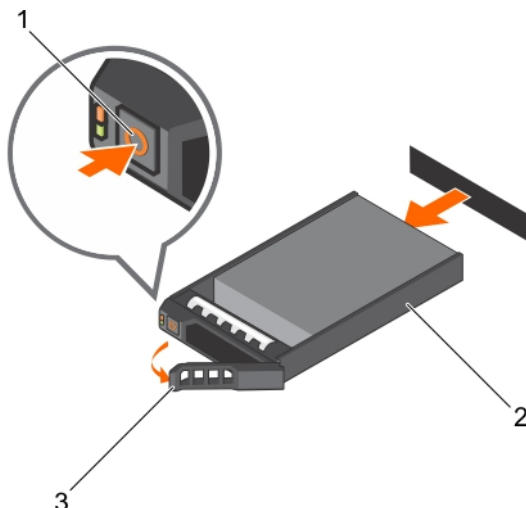
Ilustración 97. Extracción de una unidad de disco duro o SSD de intercambio directo
