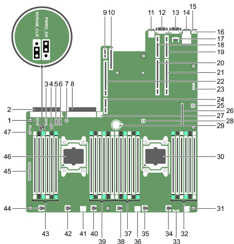
Ilustración 128. Puentes y conectores de la placa base
