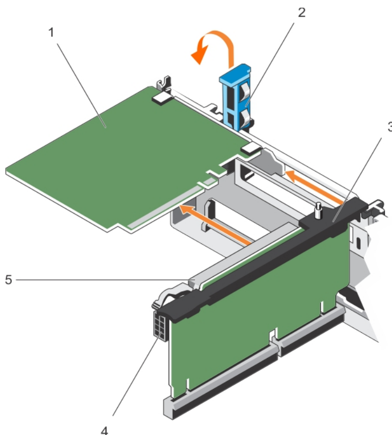
Ilustración 52. Extracción de una tarjeta de expansión del soporte vertical para tarjetas de expansión 2 o 3
