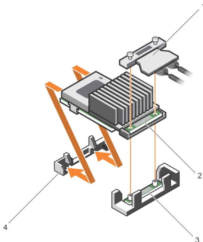
Ilustración 51. Instalación de la tarjeta controladora de almacenamiento integrada
