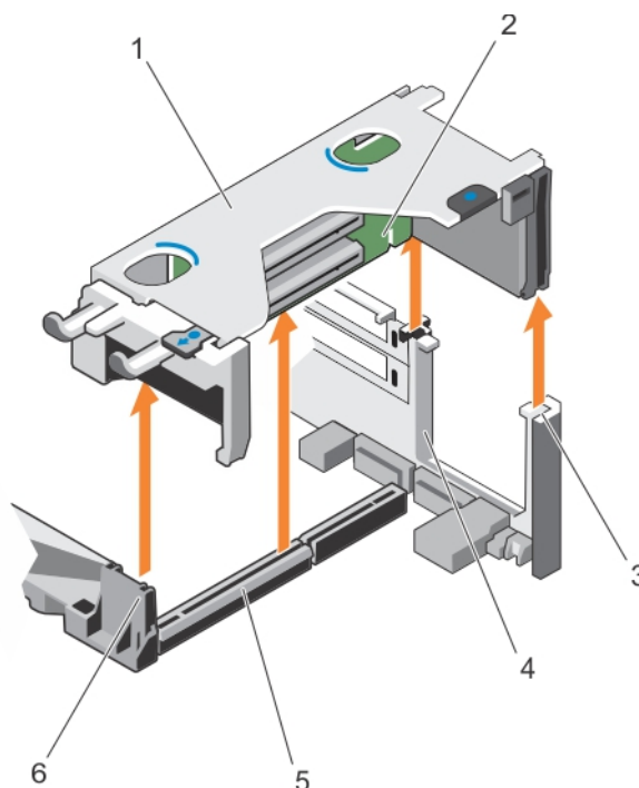
Ilustración 60. Extracción del soporte vertical para tarjetas de expansión 1
