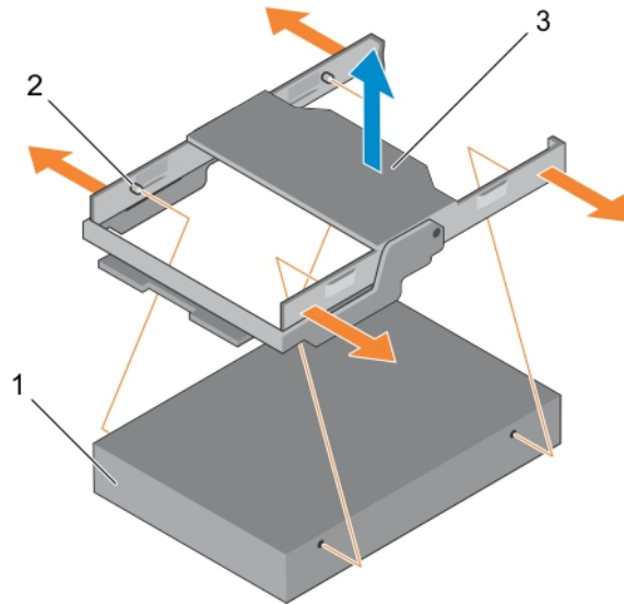
Ilustración 29. Extracción de la unidad de disco duro de un portaunidades de disco duro
