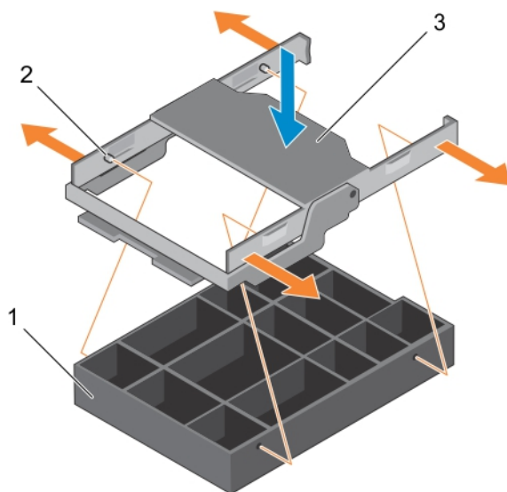
Ilustración 26. Instalación de una unidad de disco duro de relleno en un portaunidades de disco duro
