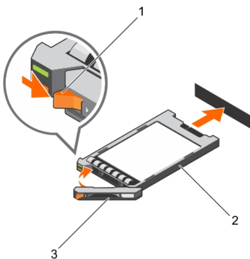
Ilustración 100. Instalación de un portaunidades de SSD uSATA de 1,8 pulgadas de intercambio directo
