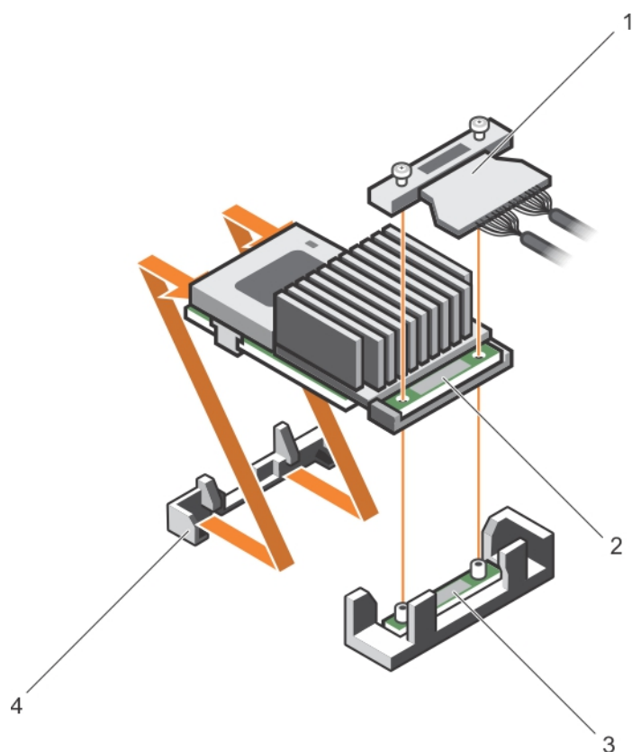
Ilustración 50. Extracción de la tarjeta controladora de almacenamiento integrada
