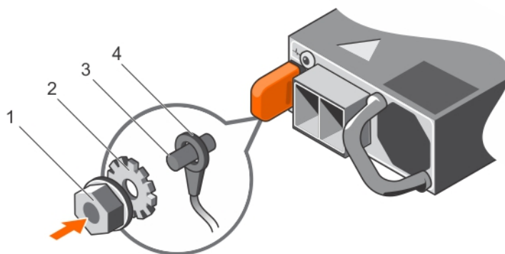
Ilustración 82. Ensamblaje y conexión del cable de toma de tierra de seguridad
