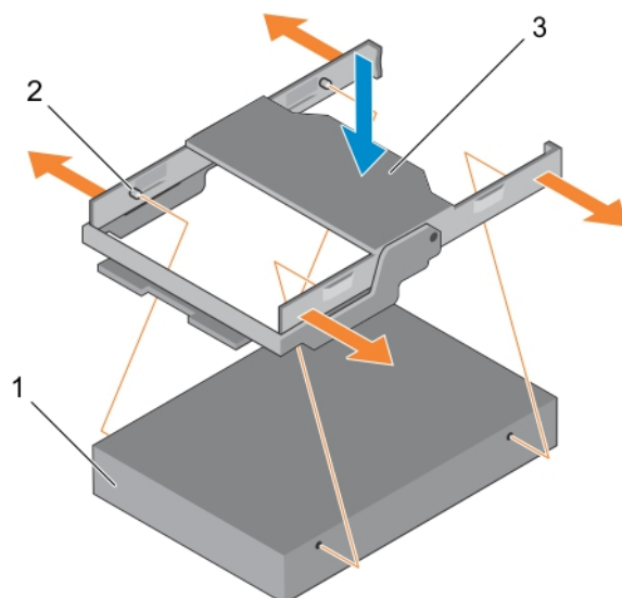
Ilustración 30. Instalación de una unidad de disco duro en un portaunidades de disco duro
