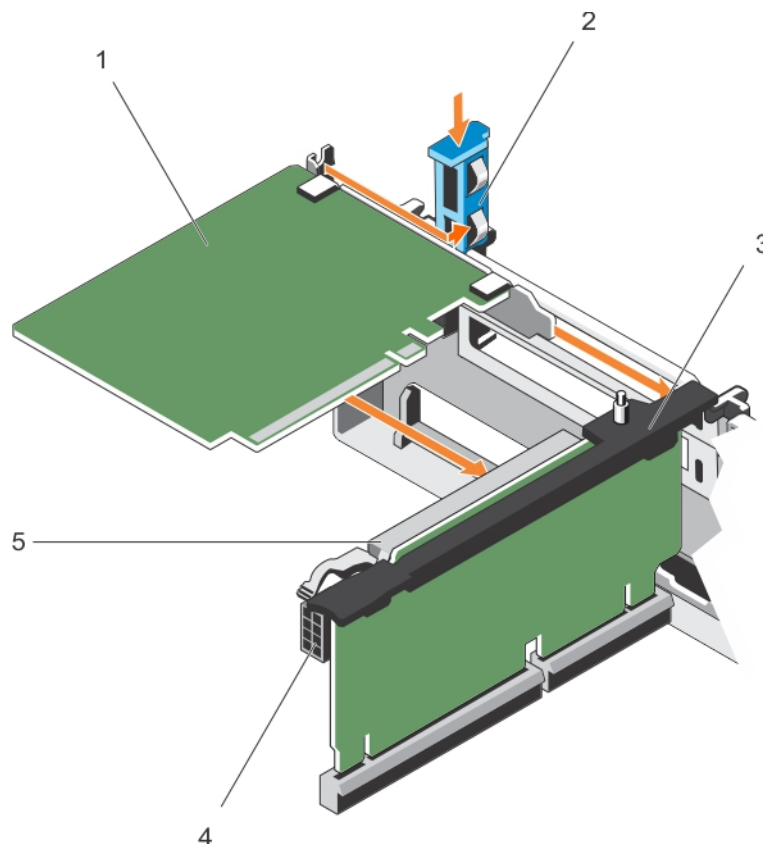
Ilustración 53. Instalación de una tarjeta de expansión en el soporte vertical para tarjetas de expansión 2 o 3
