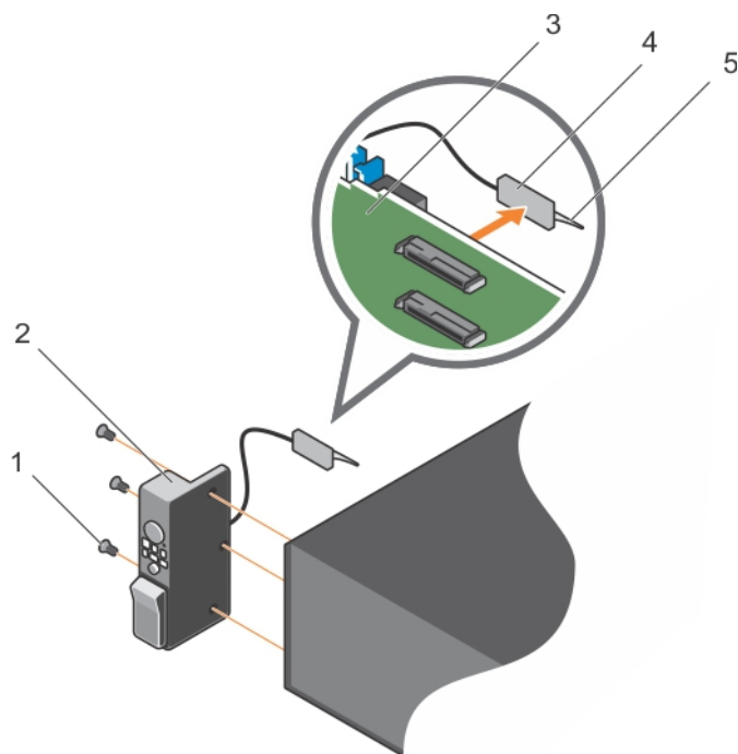
Ilustración 124. Extracción del panel de control
