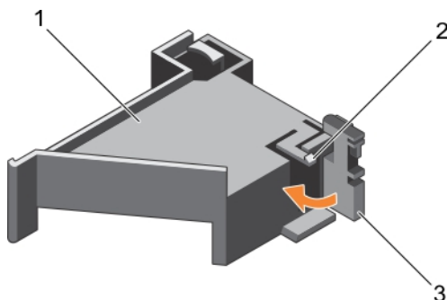
Ilustración 47. Cierre del pestillo del soporte de tarjeta PCIe
