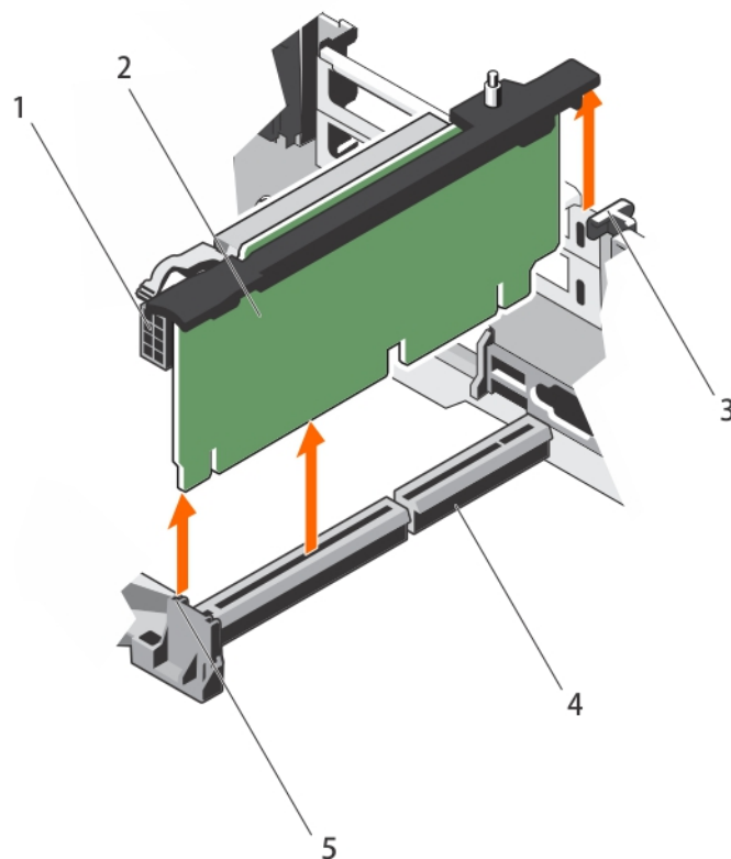
Ilustración 62. Extracción del soporte vertical para tarjetas de expansión 2
