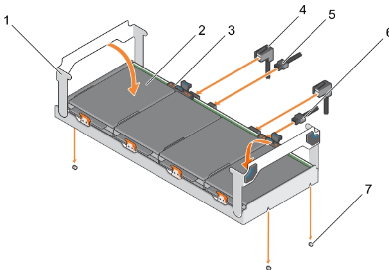
Ilustración 24. Instalación de la bandeja de la unidad de disco duro
