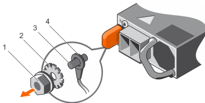
Ilustración 83. Cómo extraer el cable de toma a tierra de seguridad
