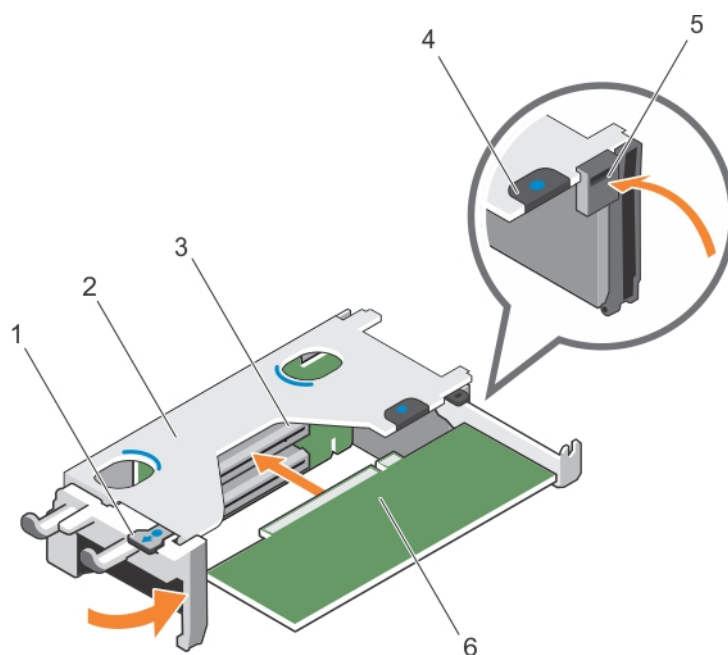
Ilustración 55. Instalación de una tarjeta de expansión en el soporte vertical para tarjetas de expansión 1
