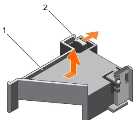
Ilustración 44. Extracción del soporte para tarjetas PCIe
