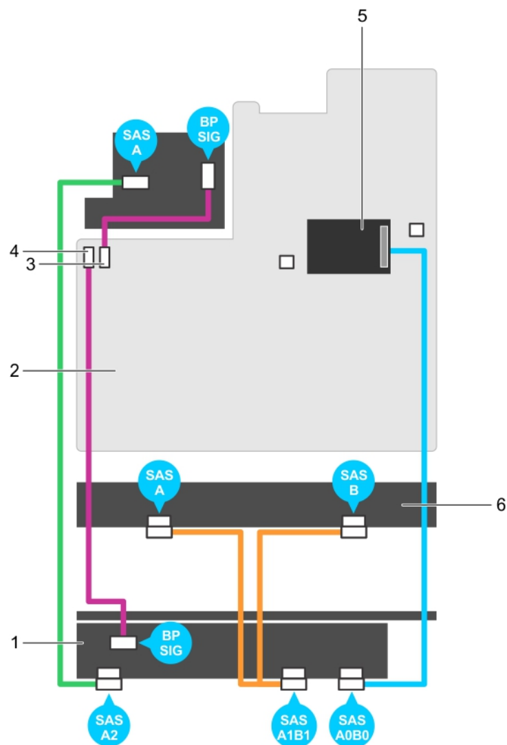
Ilustración 115. Diagrama de cableado: plano posterior SAS/SATA (x18) de 1,8 pulgadas
