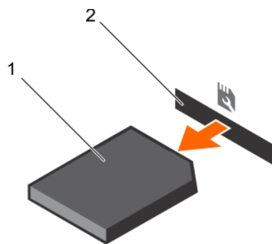
Ilustración 120. Extracción de la tarjeta multimedia vFlash SD
