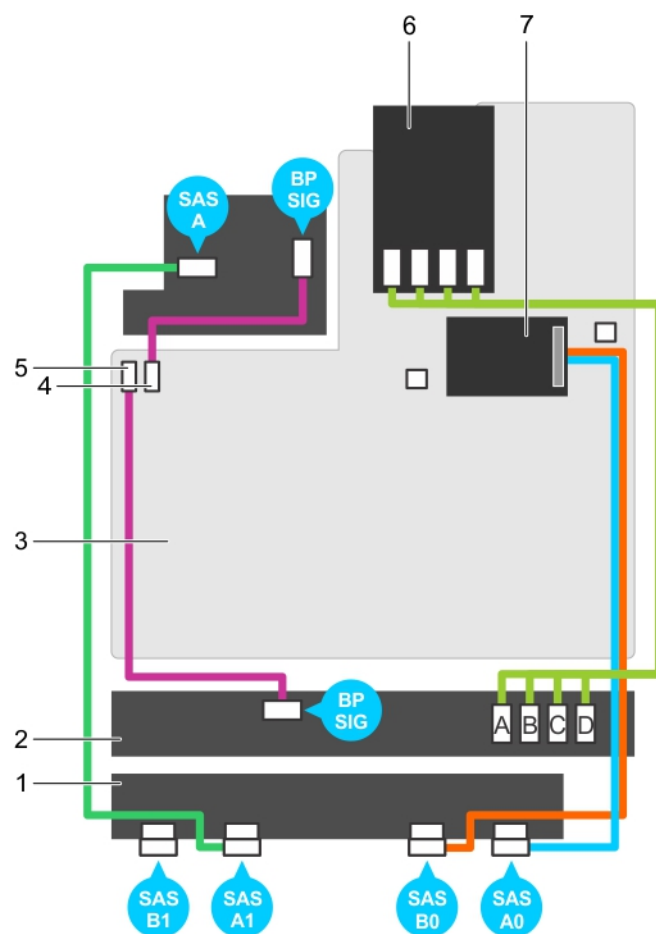
Ilustración 110. Diagrama de cableado: plano posterior SAS/SATA (x24) de 2,5 pulgadas (opción 3)
