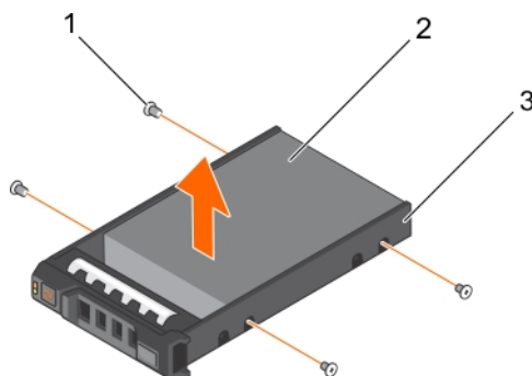
Ilustración 101. Extracción de una unidad de disco duro de un portaunidades de disco duro
