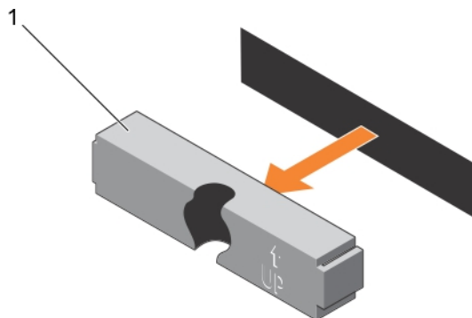
Ilustración 93. Extracción e instalación de un panel protector de unidad de disco duro de 2,5 pulgadas (parte posterior)
