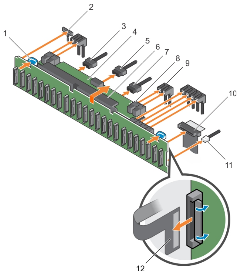
Ilustración 107. Extracción del plano posterior SAS/SATA (x24) de 2,5 pulgadas
