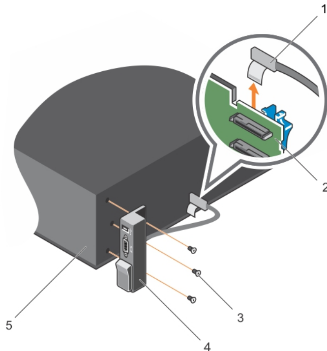
Ilustración 126. Extracción del panel de E/S
