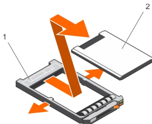
Ilustración 105. Extracción de una unidad de disco duro de 1,8 pulgadas del portaunidades de disco duro
