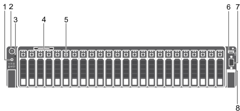
Ilustración 2. Chasis de 24 unidades de disco duro/SSD de 2,5 pulgadas
