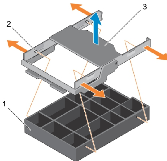
Ilustración 25. Extracción del panel protector de una unidad de disco duro de un portaunidades de disco duro
