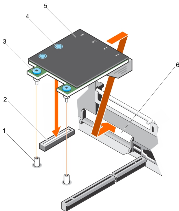
Ilustración 73. Instalación de la tarjeta NDC
