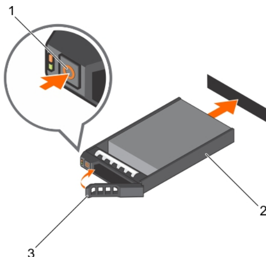
Ilustración 99. Instalación de una SSD o unidad de disco duro de intercambio directo
