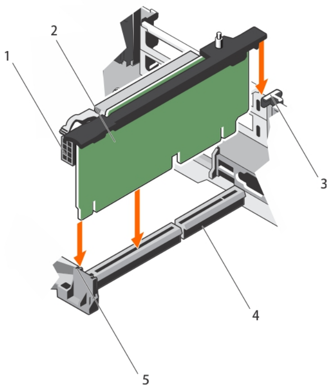
Ilustración 67. Instalación del soporte vertical para tarjetas de expansión 2
