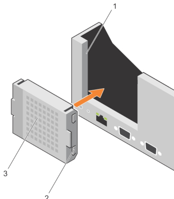
Ilustración 59. Instalación del panel de relleno de la tarjeta vertical 1
