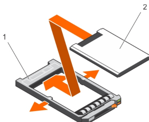
Ilustración 106. Instalación de una unidad de disco duro de 1,8 pulgadas en un portaunidades de disco duro
