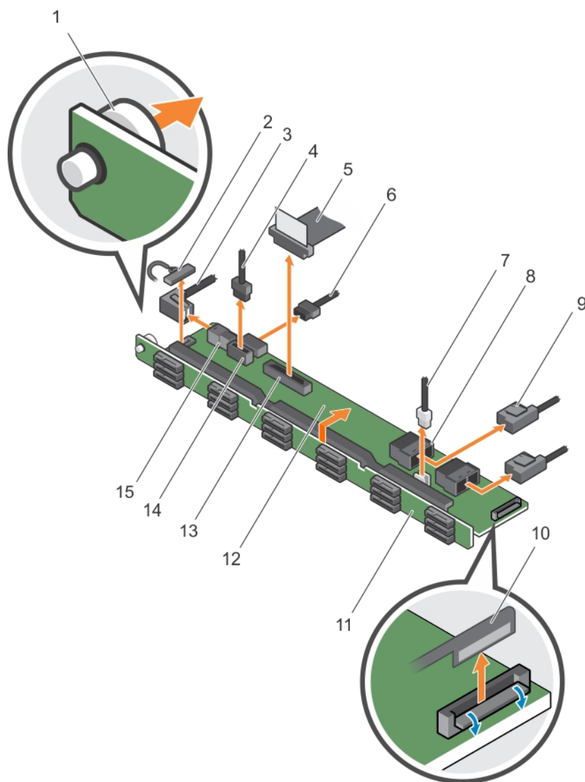
Ilustración 114. Extracción del plano posterior SAS/SATA (x18) de 1,8 pulgadas
