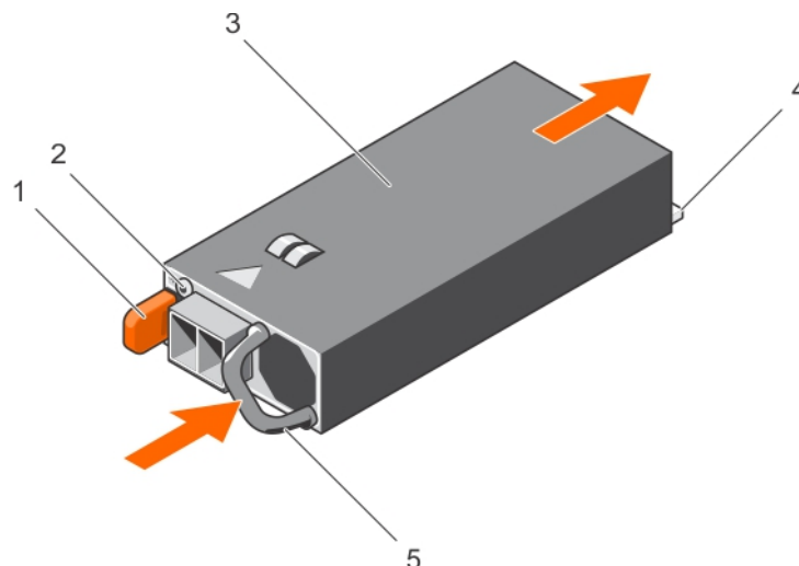
Ilustración 87. Instalación de una PSU de CC
