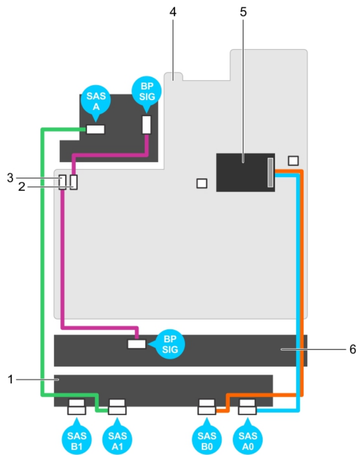
Ilustración 108. Diagrama de cableado: plano posterior SAS/SATA (x24) de 2,5 pulgadas (opción 1)
