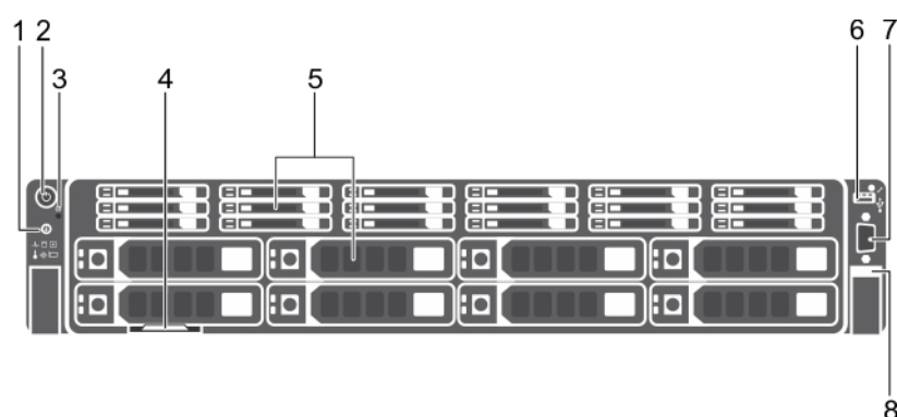
Ilustración 4. 8 chasis de unidad de disco duro de 3,5 pulgadas y 18 chasis de SSD de 1,8 pulgadas
