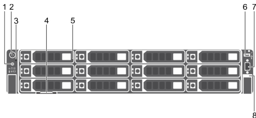
Ilustración 3. 12 chasis de unidad de disco duro de 3,5 pulgadas
