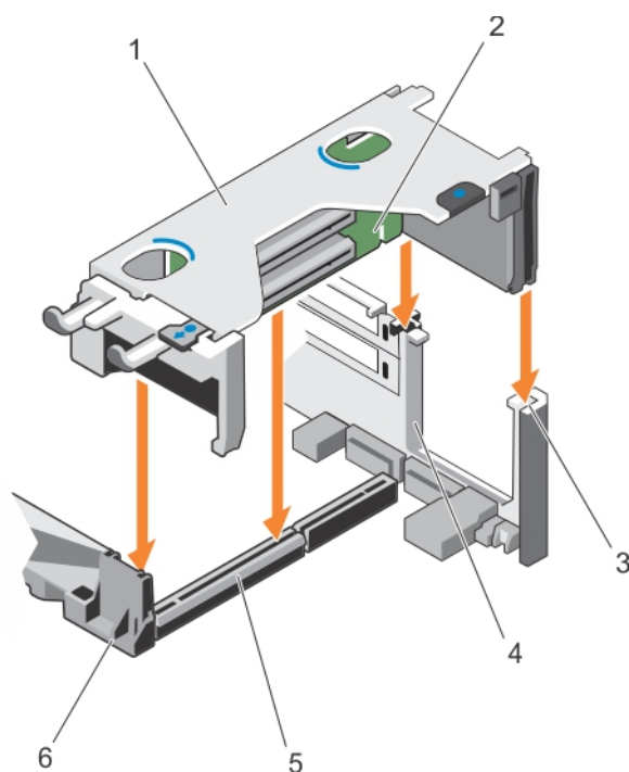
Ilustración 66. Instalación del soporte vertical para tarjetas de expansión 1
