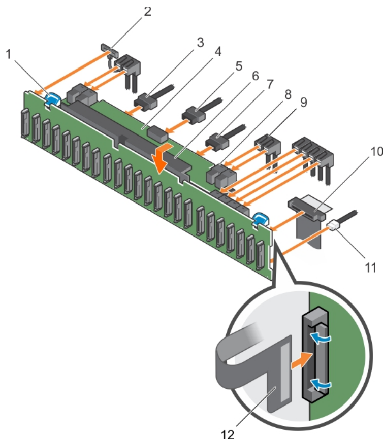
Ilustración 116. Instalación del plano posterior SAS/SATA (x24) de 2,5 pulgadas
