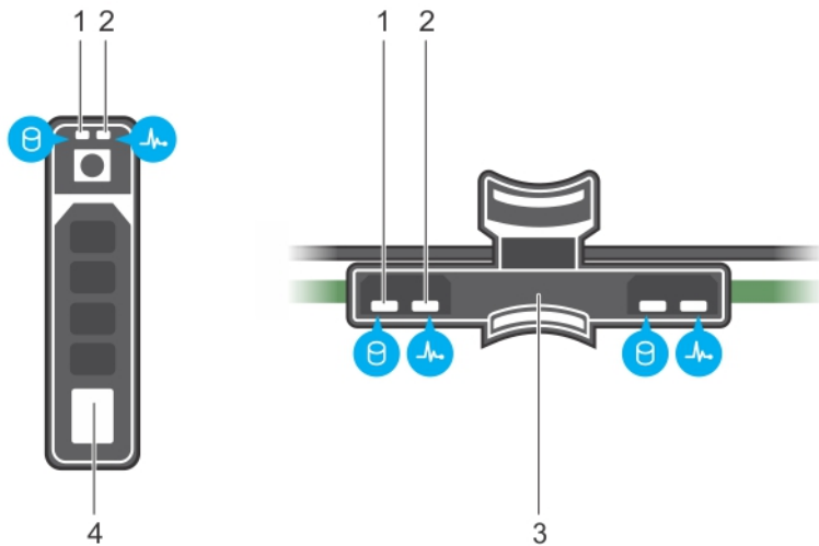
Ilustración 6. Indicadores de la unidad de disco duro en la unidad de disco duro y en el plano posterior de la bandeja de la unidad de disco duro
