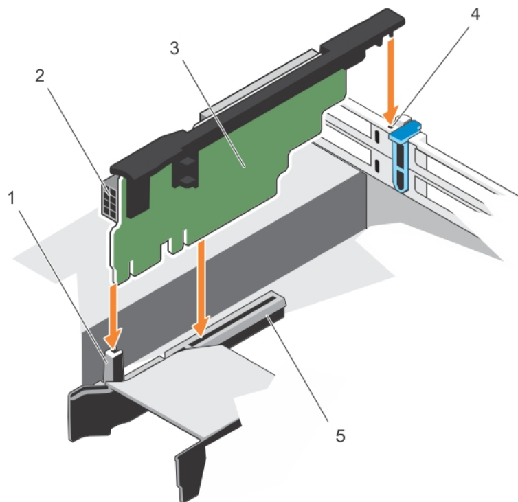
Ilustración 68. Instalación del soporte vertical para tarjetas de expansión 3
