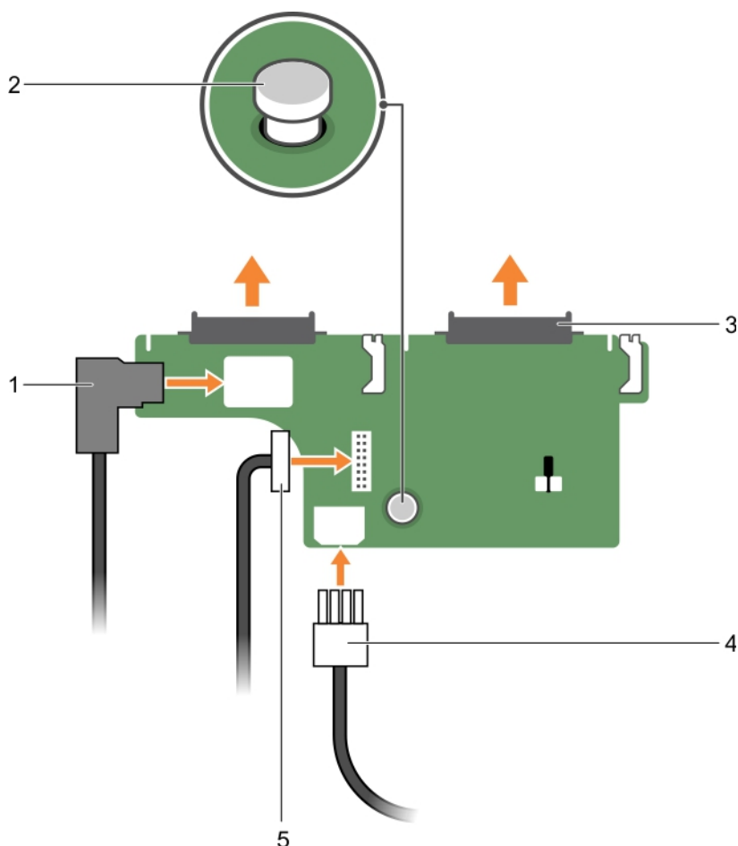
Ilustración 119. Instalación del plano posterior de la unidad de disco duro de 2,5 pulgadas (x2) opcional
