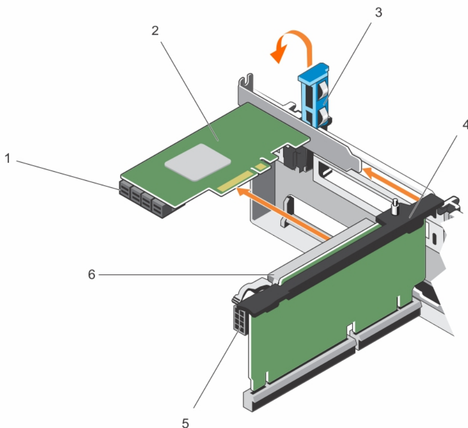
Ilustración 56. Extracción de una tarjeta de expansión de NVMe del soporte vertical para tarjetas de expansión
