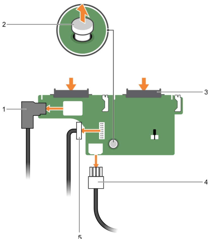
Ilustración 118. Extracción del plano posterior de la unidad de disco duro de 2,5 pulgadas (x2) opcional
