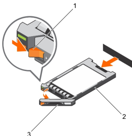
Ilustración 98. Extracción de un portaunidades de SSD uSATA de 1,8 pulgadas de intercambio activo
