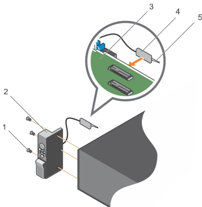
Ilustración 125. Instalación del panel de control
