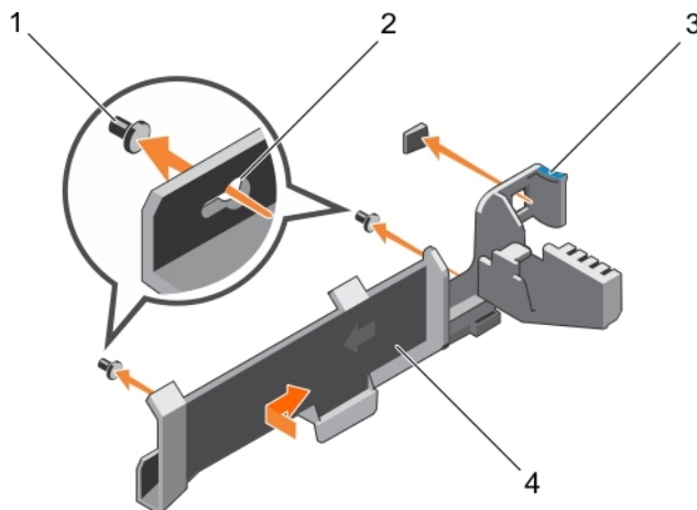
Ilustración 49. Instalación del soporte de retención de cables
