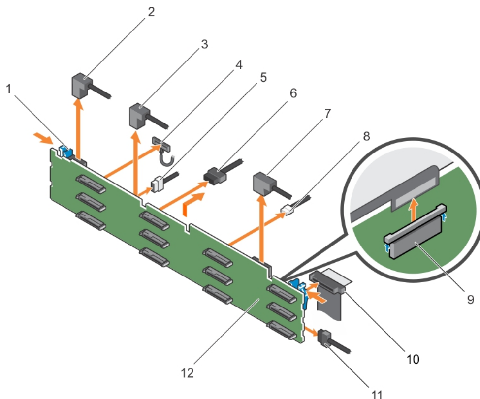
Ilustración 111. Extracción del backplane de SAS/SATA de 3.5 pulgadas (x12)
