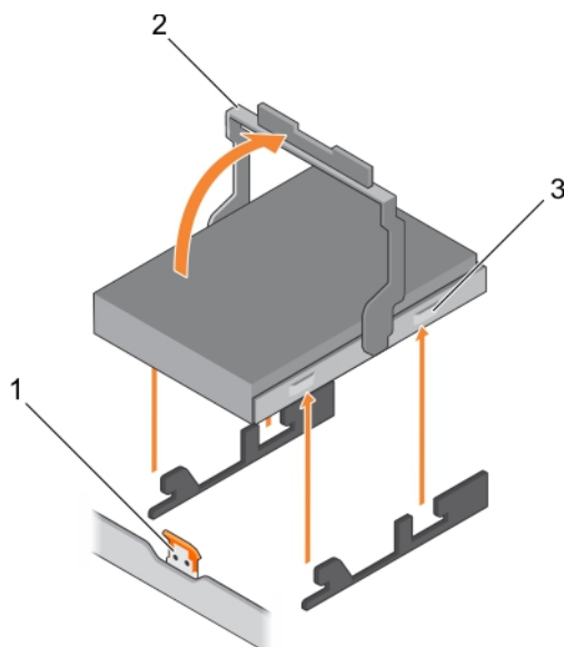
Ilustración 27. Extracción de una unidad de disco duro de la bandeja de la unidad de disco duro
