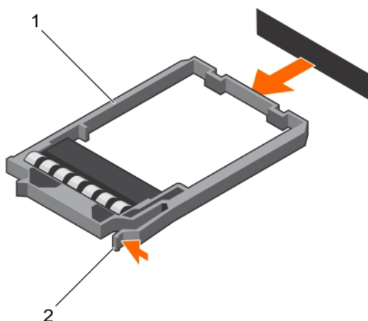
Ilustración 103. Extracción de una unidad de disco duro de relleno de 1,8 pulgadas
