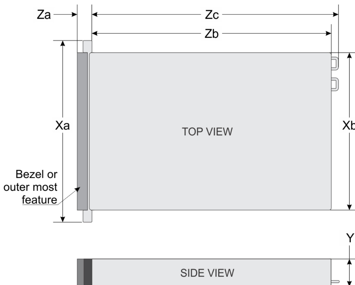
Ilustración 13. Dimensiones del chasis del sistema Dell PowerEdge R730xd
