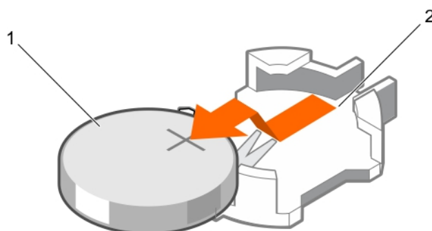
Ilustración 76. Extracción de la batería del sistema
