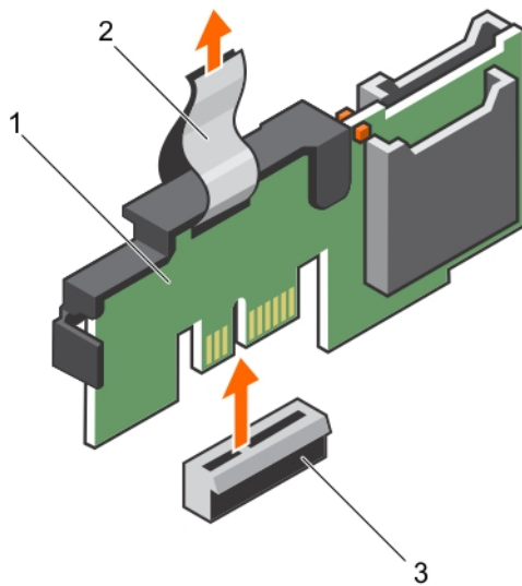
Ilustración 71. Extracción del módulo SD dual interno (IDSDM)
