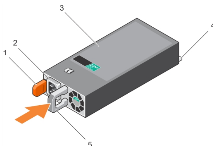
Ilustración 81. Instalación de una unidad de fuente de alimentación de CA
