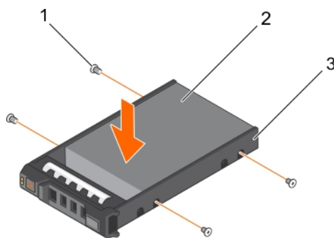
Ilustración 102. Instalación de una unidad de disco duro en un portaunidades de disco duro
