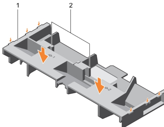
Ilustración 22. Instalación de la cubierta de refrigeración
