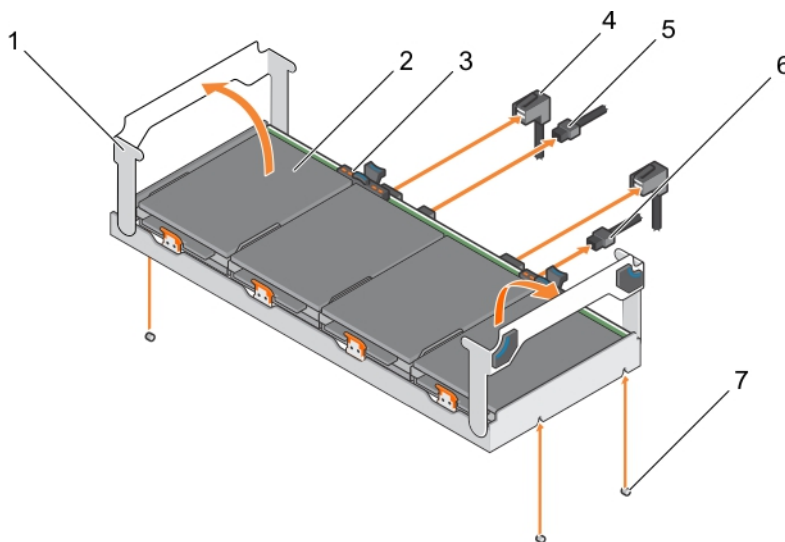
Ilustración 23. Extracción de la bandeja de la unidad de disco duro
