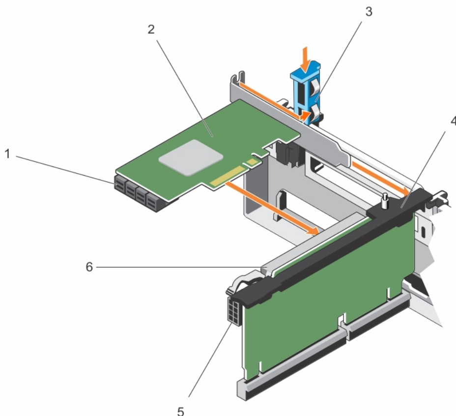
Ilustración 57. Instalación de una tarjeta de expansión en el soporte vertical para tarjetas de expansión
