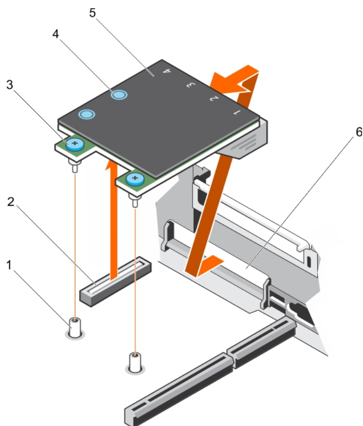
Ilustración 72. Extracción de la tarjeta NDC
