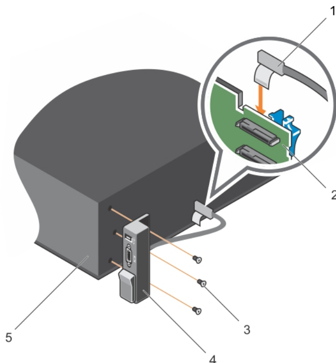
Ilustración 127. Instalación del panel de E/S
