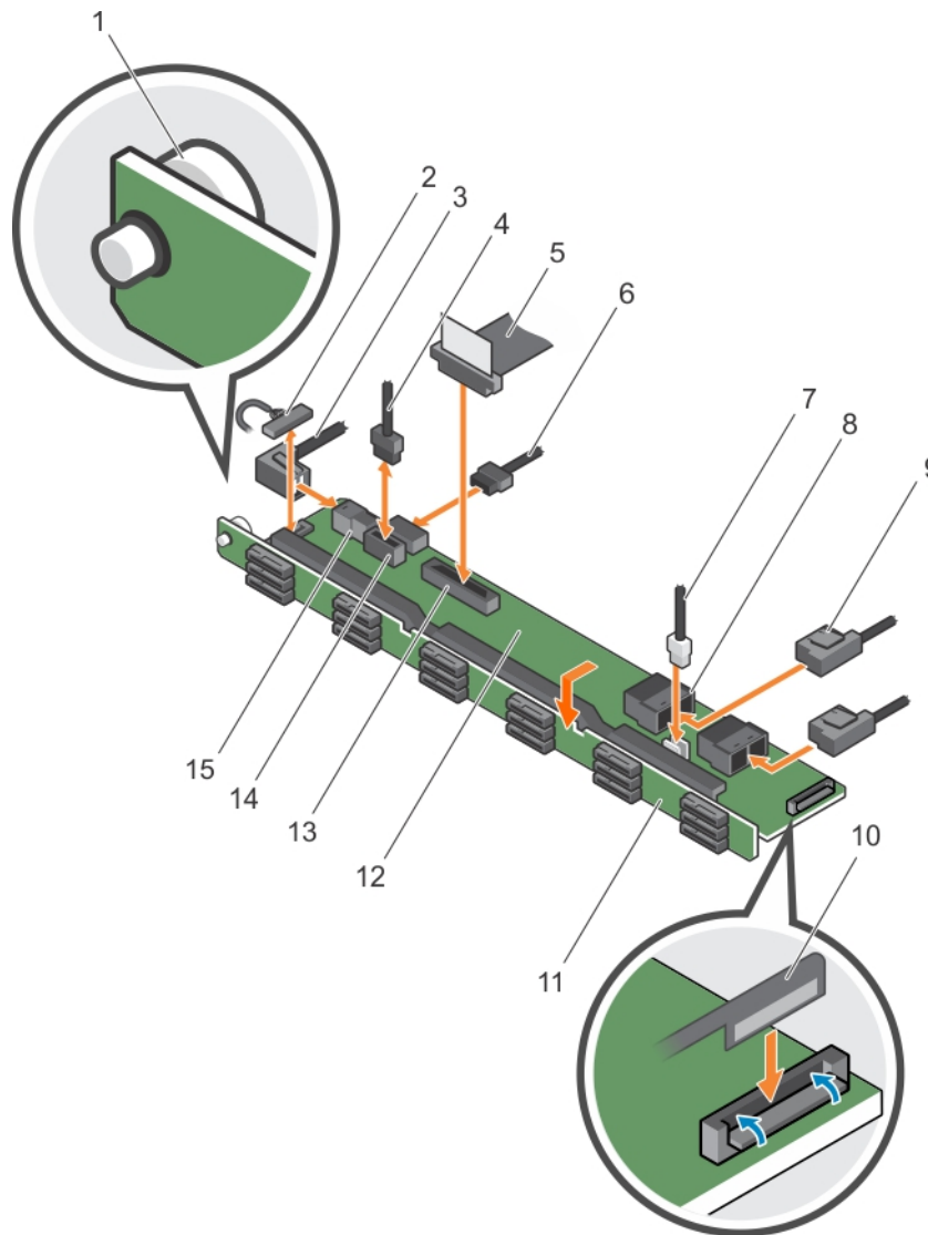
Ilustración 117. Instalación del plano posterior SAS/SATA (x18) de 1,8 pulgadas
