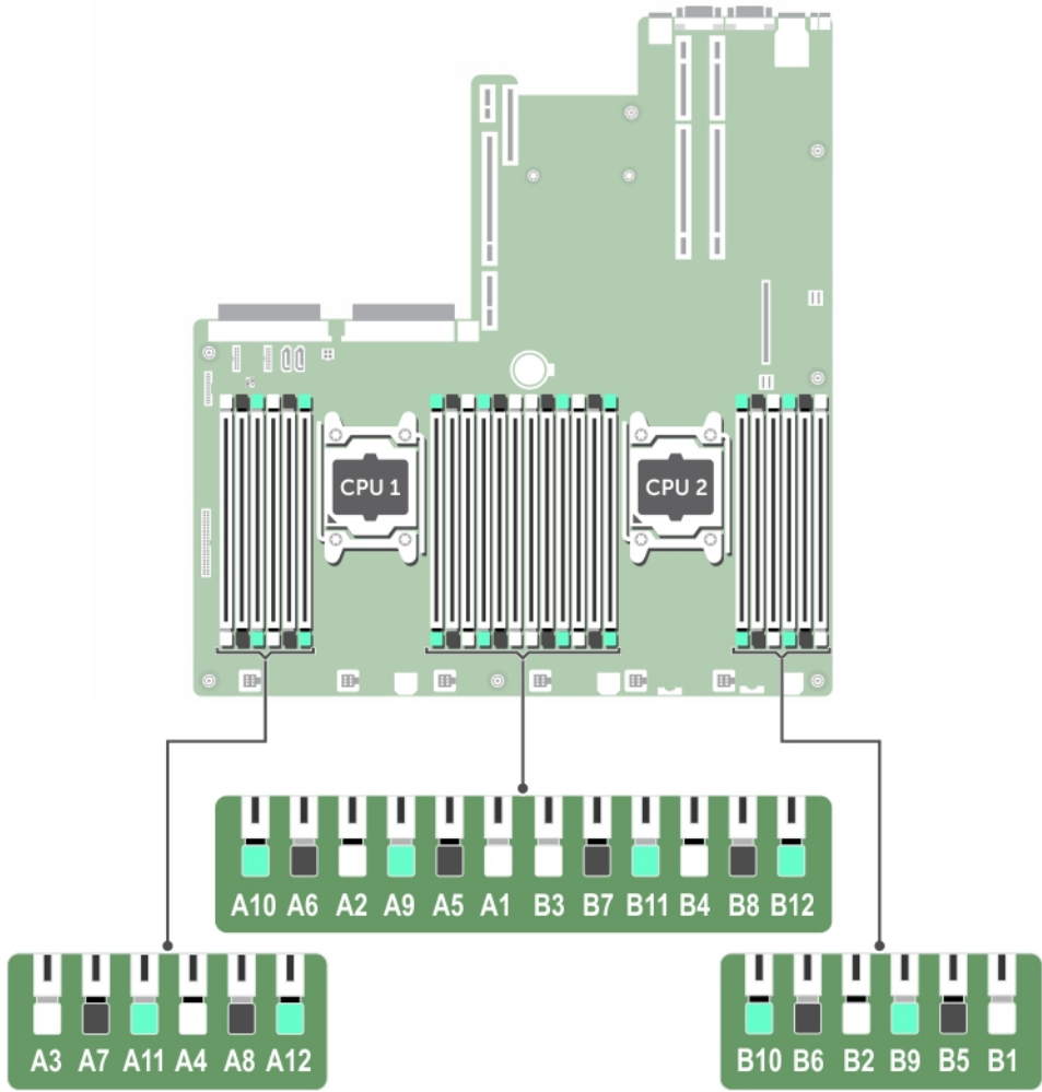
Ilustración 35. Ubicaciones de los sockets de memoria
