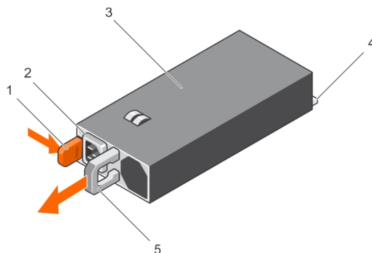
Ilustración 80. Extracción de una unidad de fuente de alimentación de CA
