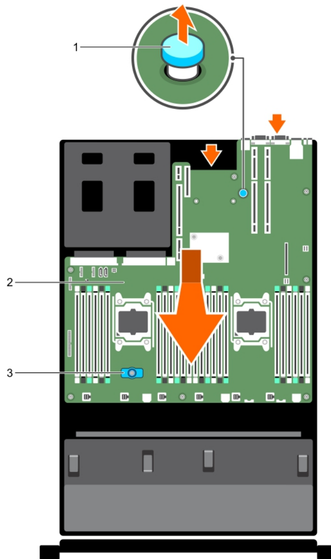
Ilustración 88. Extracción de la placa base
