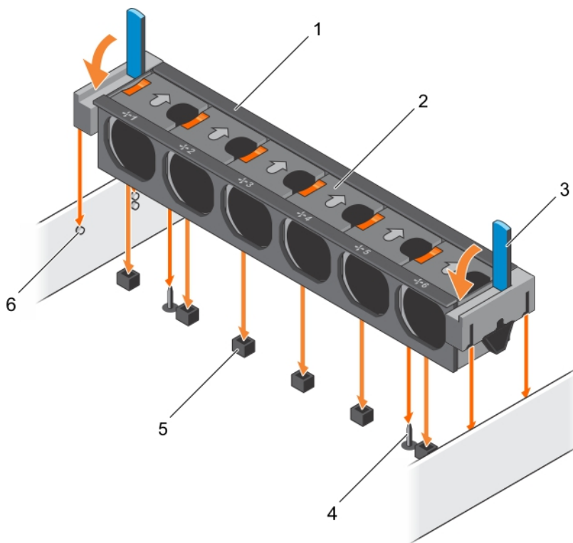
Ilustración 34. Instalación del ensamblaje de ventiladores
