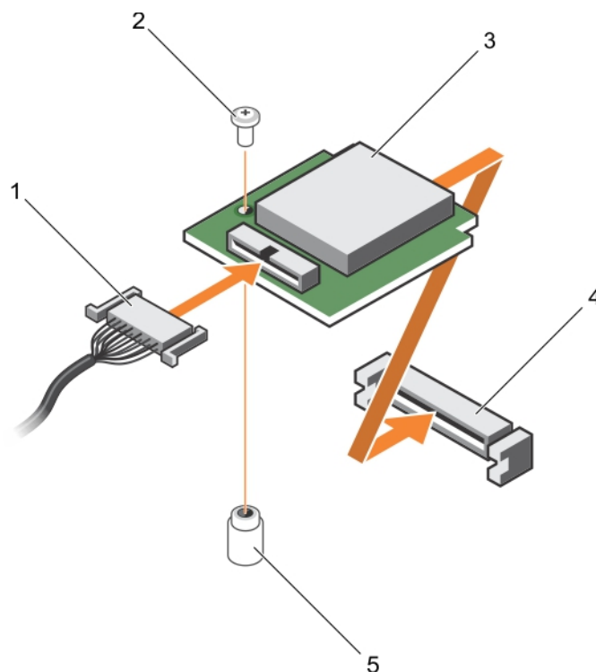
Ilustración 123. Instalación de una unidad de memoria vFlash
