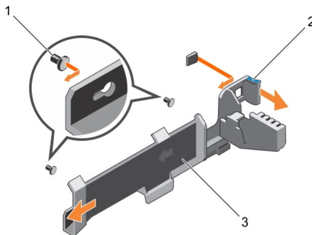
Ilustración 48. Extracción del soporte de retención de cables
