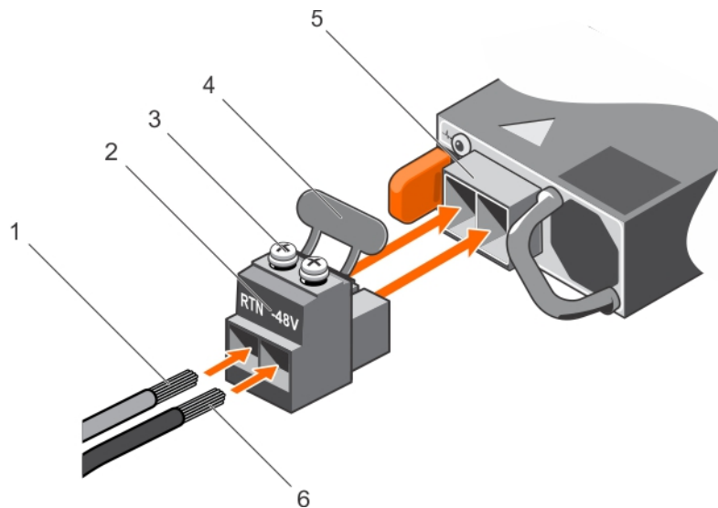
Ilustración 84. Ensamblaje de los cables de alimentación de entrada de CC
