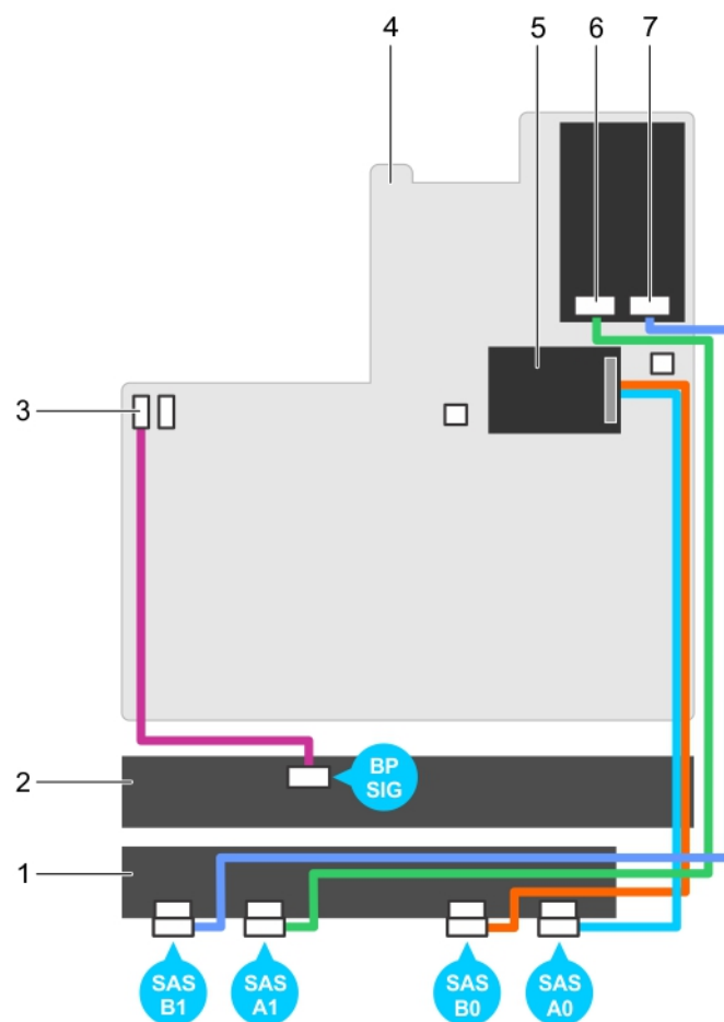
Ilustración 109. Diagrama de cableado: plano posterior SAS/SATA (x24) de 2,5 pulgadas (opción 2)
