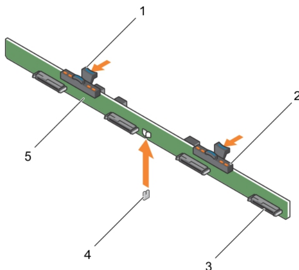
Ilustración 31. Extracción del plano posterior de la unidad de disco duro de 3,5 pulgadas (x4)
